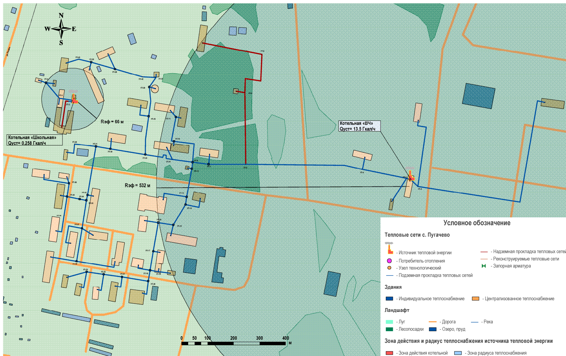
Рис. 3.1. Схема с обозначением радиуса эффективного теплоснабжения источника тепловой энергии – котельная «Войсковая Часть» и «Школьная» с. Пугачево.
