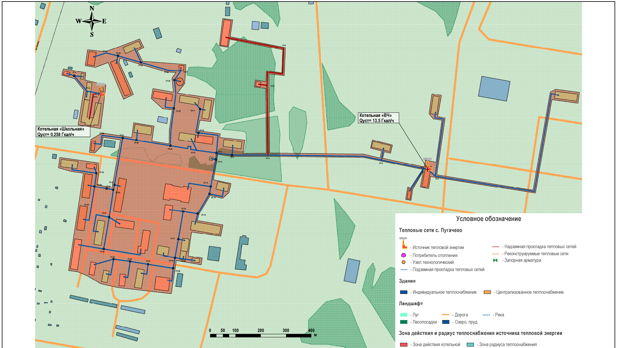
Рисунок 3.2. Существующая зона действия системы теплоснабжения и источника тепловой энергии – котельная «Войсковая Часть» и «Школьная» с. Пугачево.
