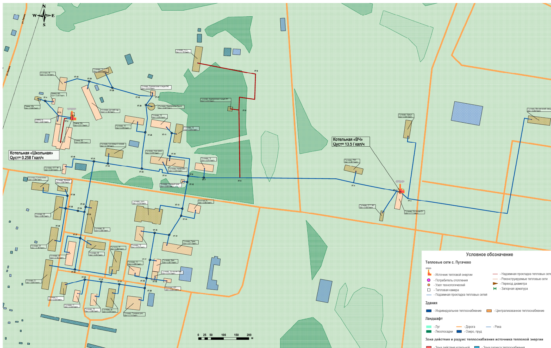
Рис. 1.2. Принципиальная схема места расположения источника тепловой энергии – котельная «Войсковая Часть» с. Пугачево
