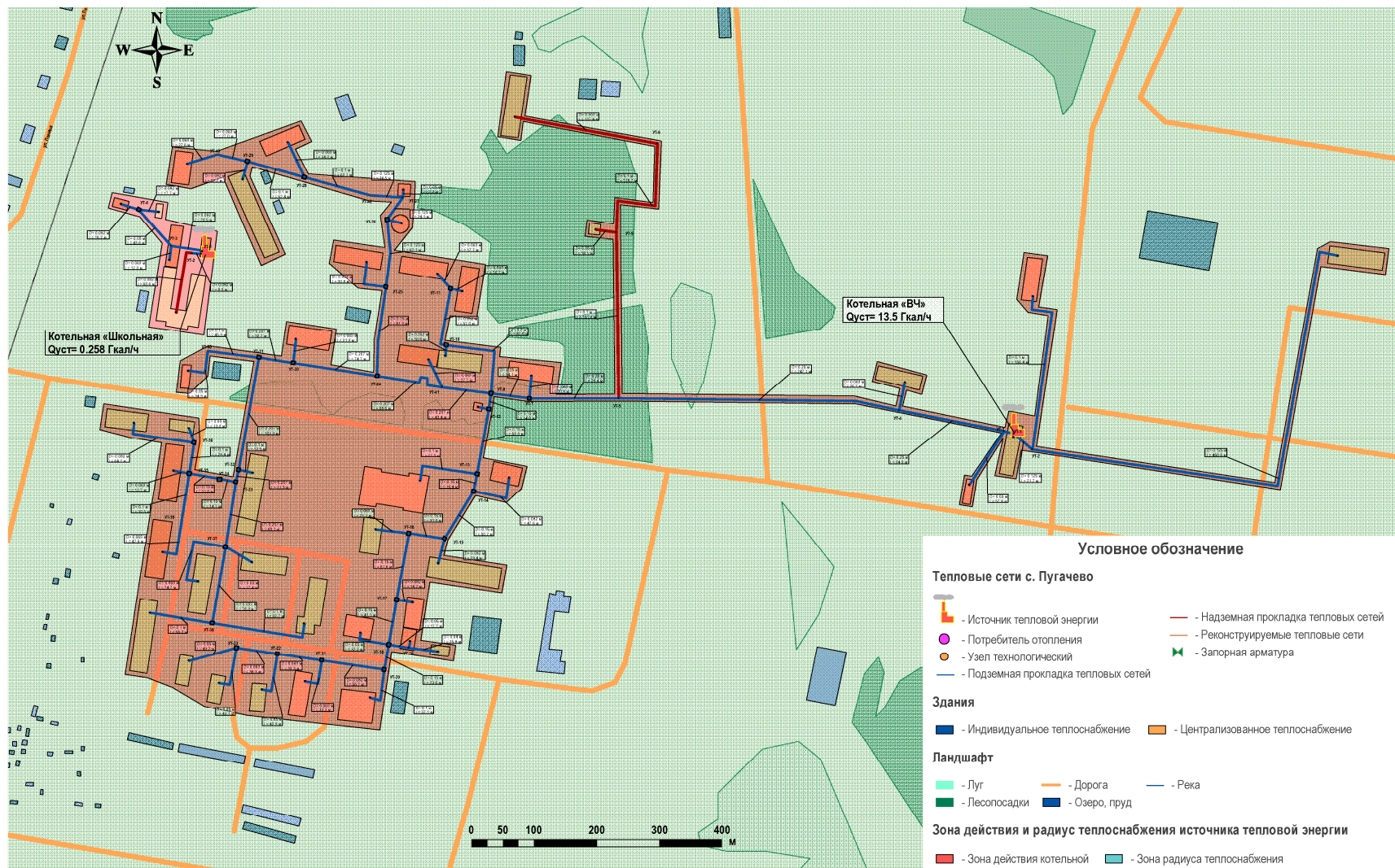
Рис. 4.2. Перспективная зона действия системы теплоснабжения и источников тепловой энергии – котельная «Войсковая Часть» и котельная «Школьная» с. Пугачево.
