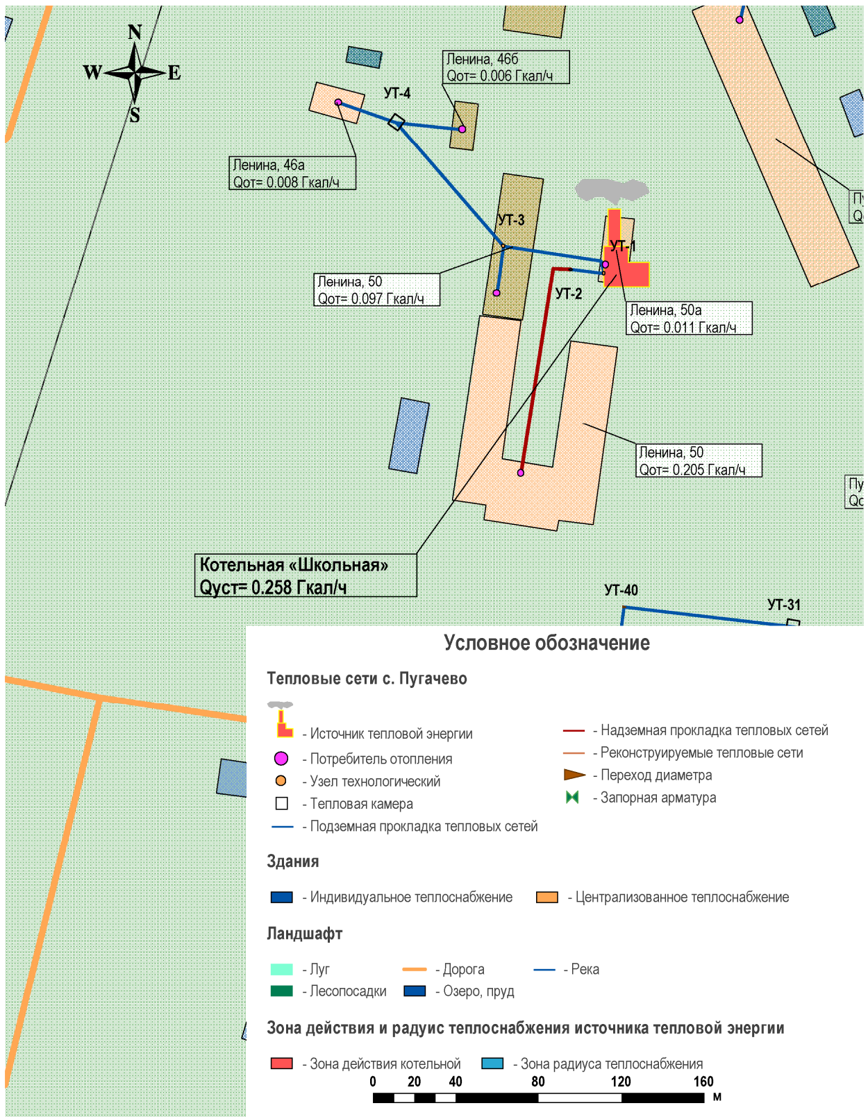
Рис. 1.3. Принципиальная схема места расположения источника тепловой энергии – котельная «Школьная» с. Пугачево.
