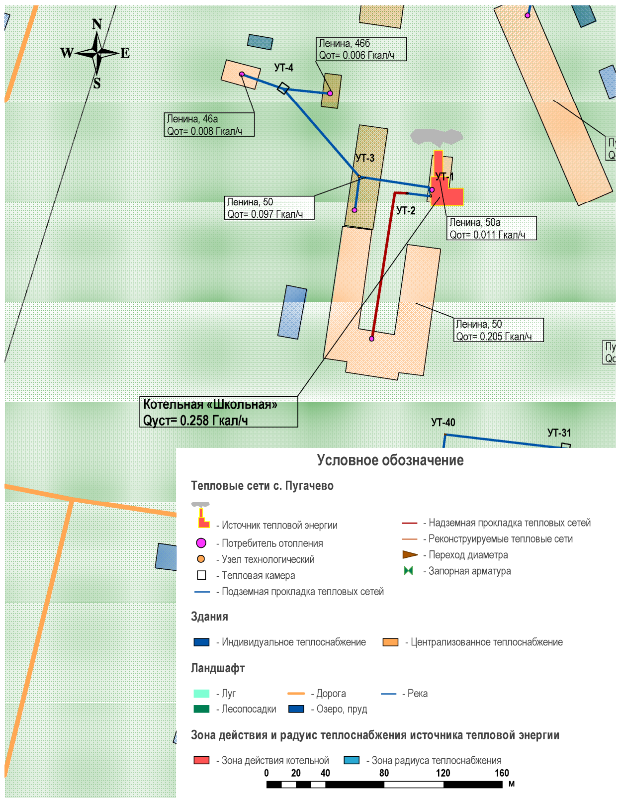
Рис. 2.2. Схема с указанием объемов потребления тепловой энергии от котельной «Школьная» с. Пугачево.
