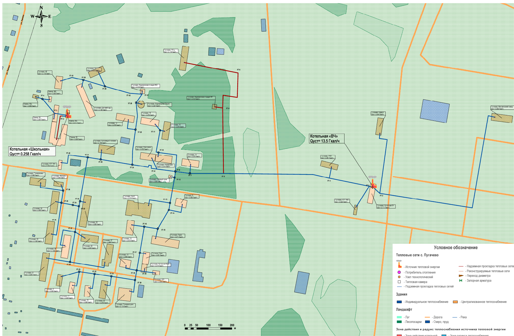
Рис. 2.1. Схема с указанием объемов потребления тепловой энергии от котельной «Войсковая Часть» с. Пугачево.
