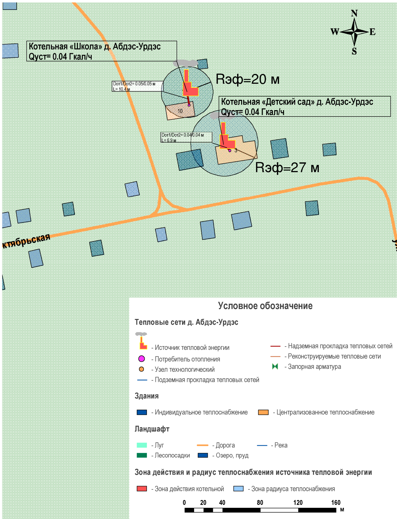
Рис. 3.3. Схема с обозначением радиуса эффективного теплоснабжения источников тепловой энергии – котельные «Школа» и «Детский сад» д. Абдэс-Урдэс.
