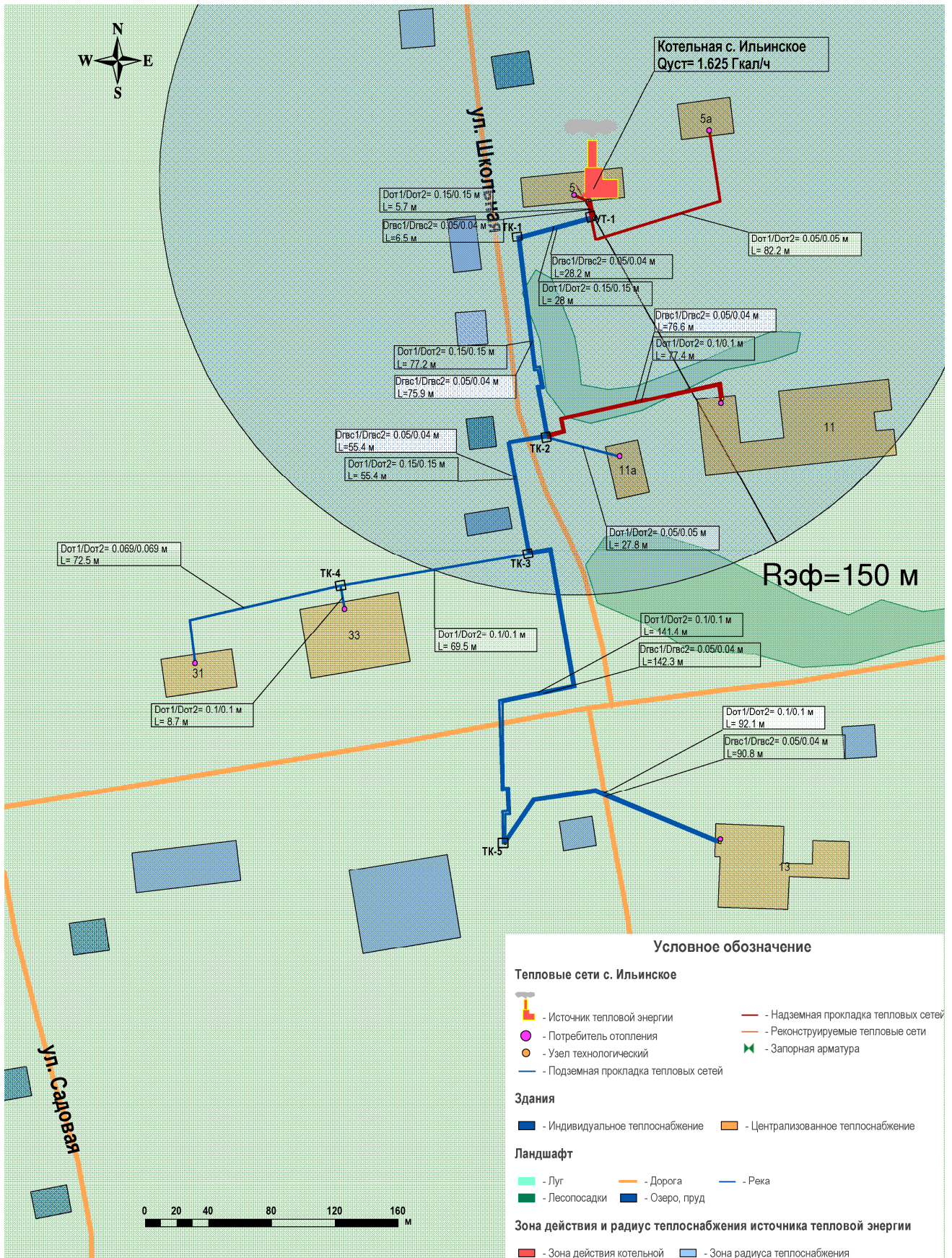
Рис. 3.2. Схема с обозначением радиуса эффективного теплоснабжения источника тепловой энергии – котельная с. Ильинское.
