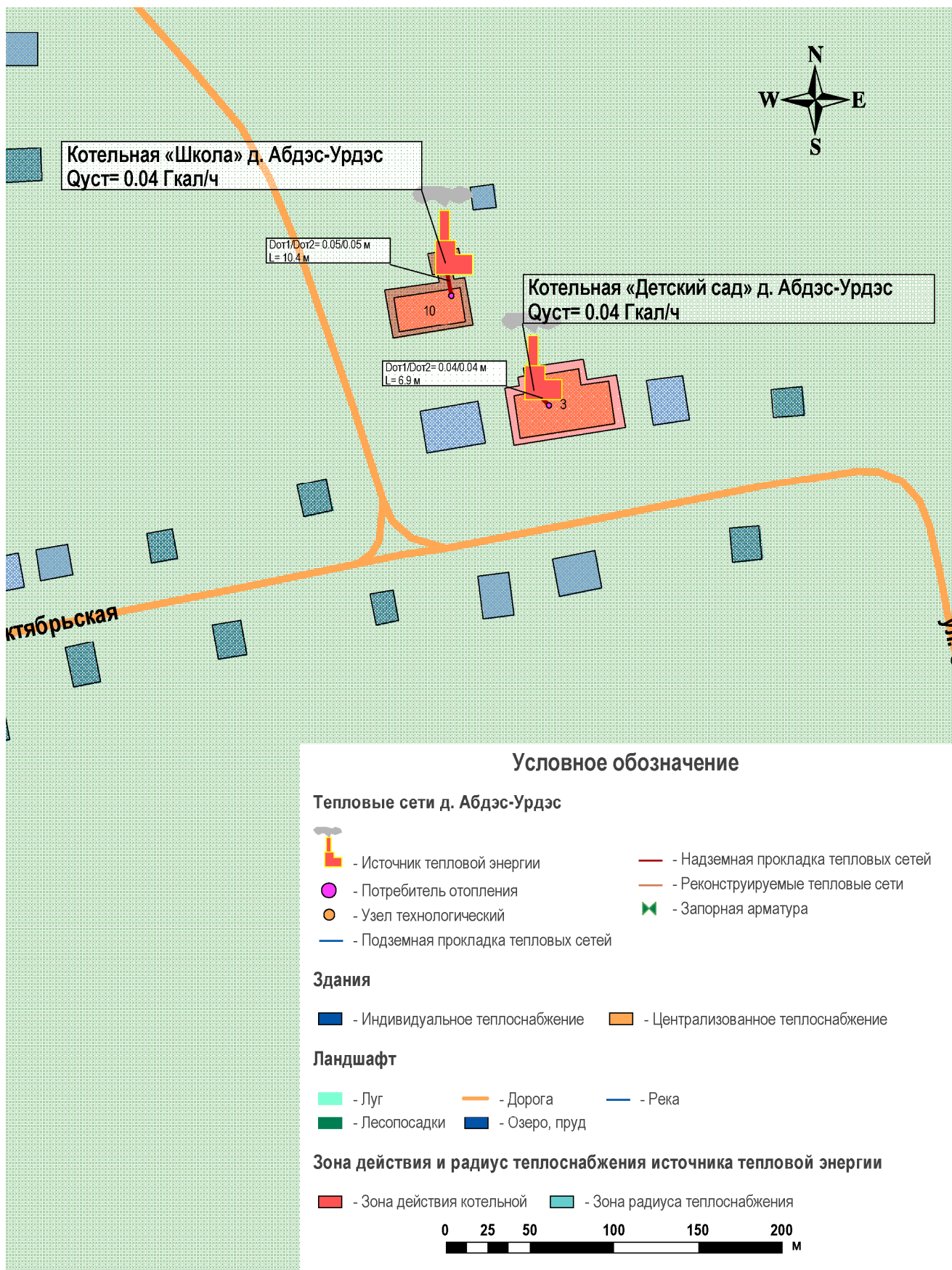
Рис. 3.5. Существующая зона действия системы теплоснабжения и источников тепловой энергии – котельные «Школа» и «Детский сад» д. Абдэс-Урдэс.
