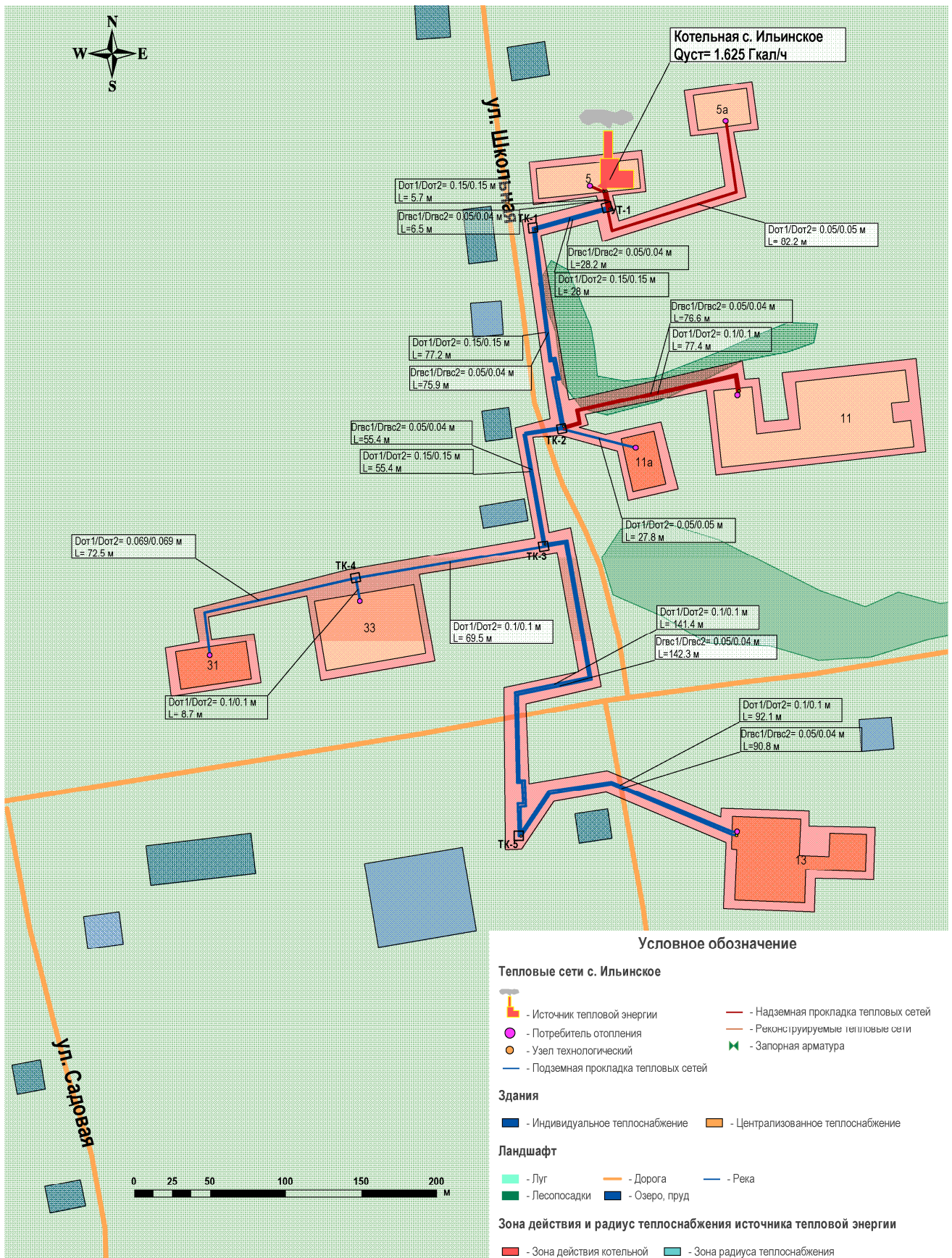
Рис. 3.4. Существующая зона действия системы теплоснабжения и источника тепловой энергии – котельная с. Ильинское.
