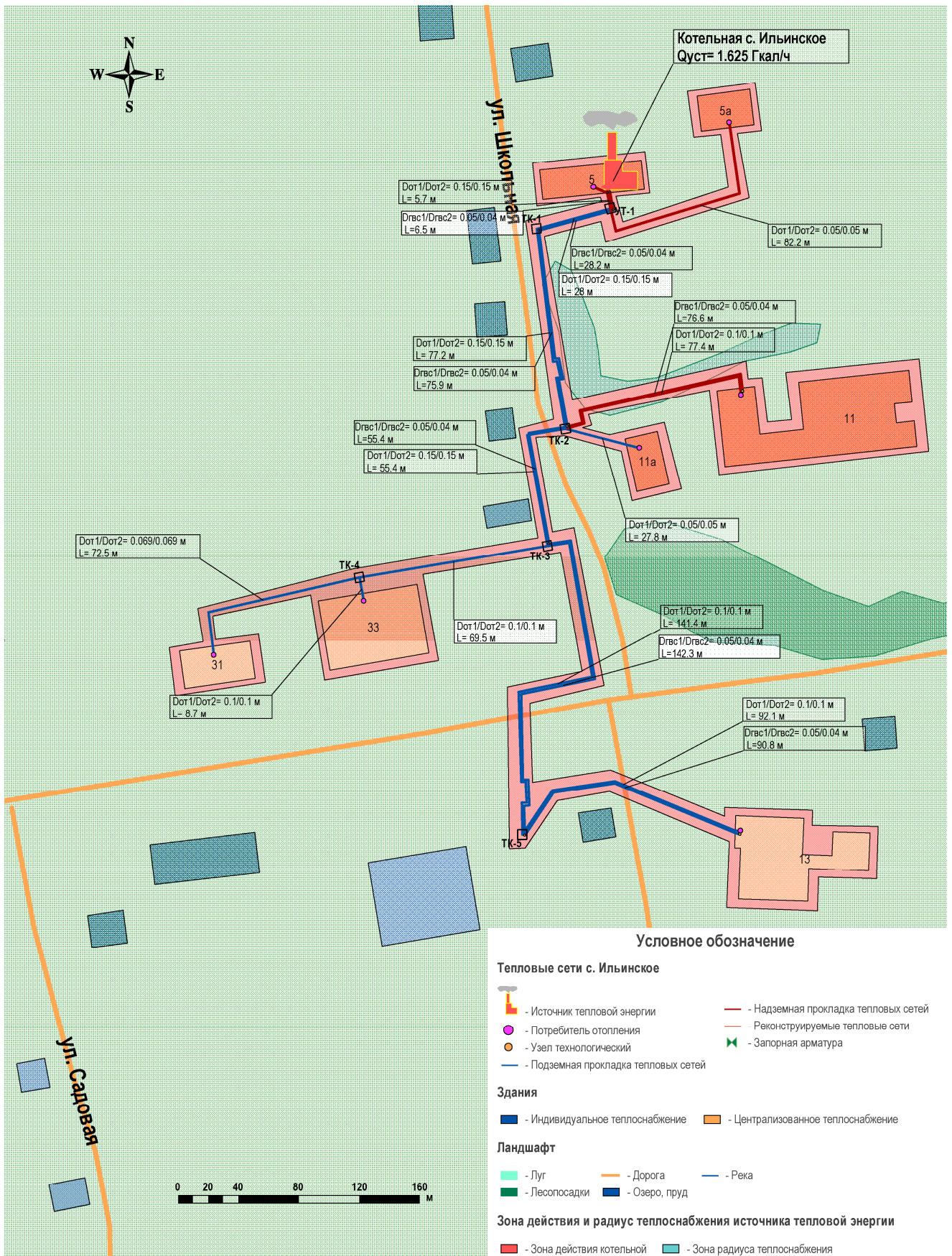
Рис. 4.2. Перспективная зона действия системы теплоснабжения и источника тепловой энергии – котельная с. Ильинское.
