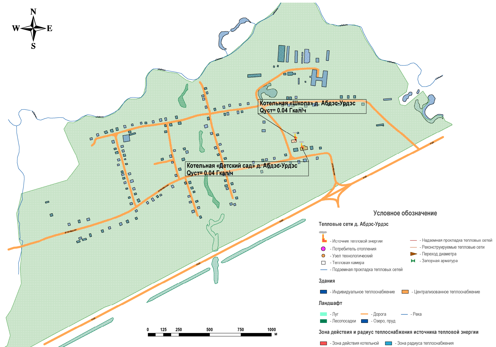
Рис. 1.2. Принципиальная схема места расположения источников тепловой энергии – котельные д. Абдэс-Урдэс.
