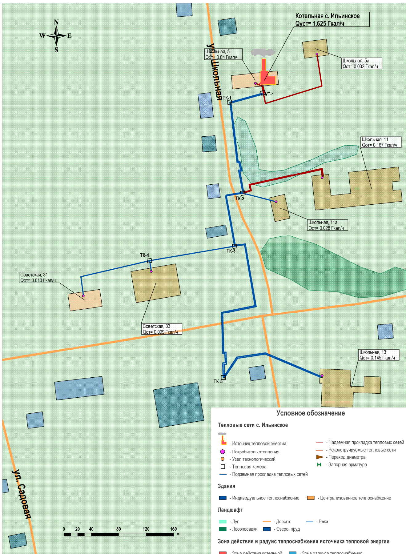
Рис. 2.1. Схема с указанием объемов потребления тепловой энергии от котельной с. Ильинское.
